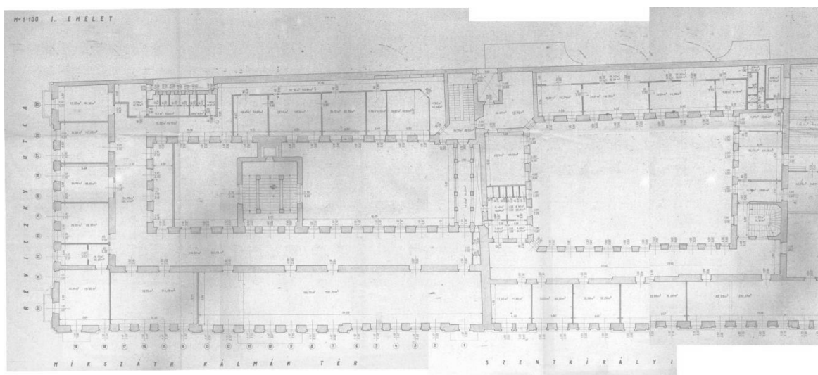
10. ábra Egykori Sophianum épületének I. emeleti vázrajza. 1951.
